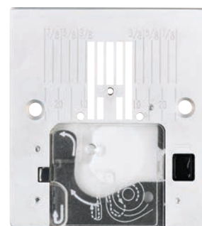
Plaque à aiguille pour point droit avec repères en pouce 820999096 quilt ambition™ 2.0 ambition™ 1.5, 1.0 ambition essential
