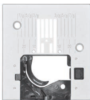
Plaque à aiguille pour point droit avec repères en pouce 821036096 passport™ 2.0, 3.0
